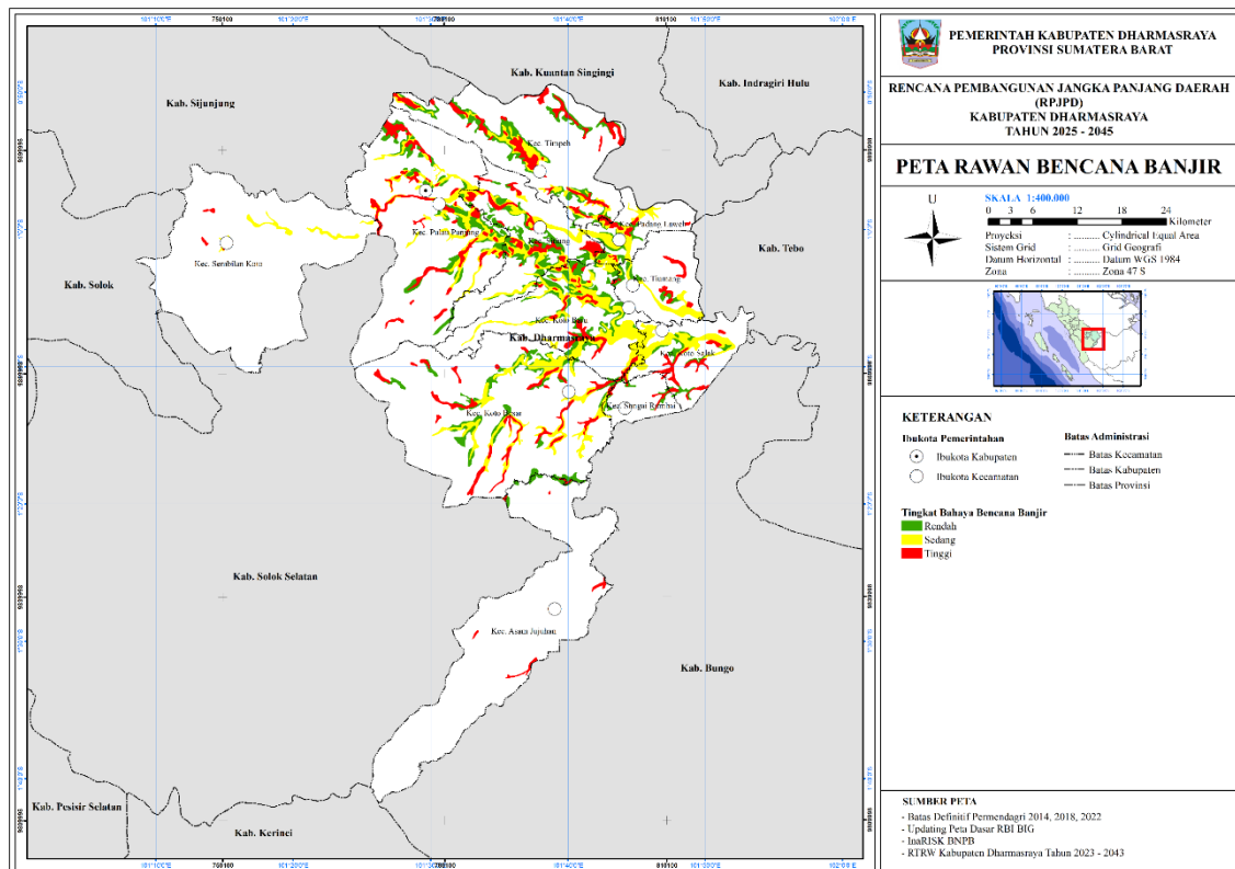
Gambar 2-10 Peta Rawan Bencana Banjir di Kabupaten Dharmasraya
