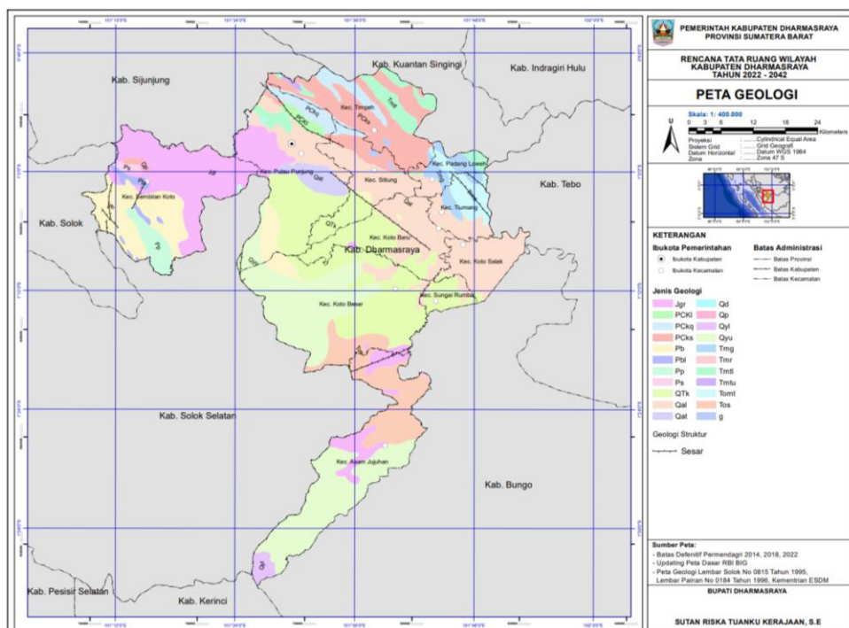
Gambar 2-5 Peta Geologi Kabupaten Dharmasraya
