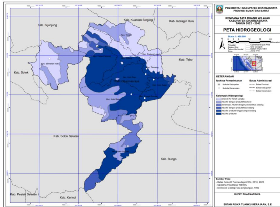
Gambar 2-6 Peta Hidrogeologi Kabupaten Dharmasraya
